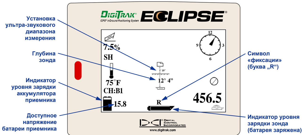
Экран индикации глубины
