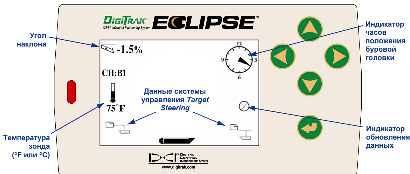
Экран дистанционного дисплея (приемник находится над передней или задней точкой или на линии локации)
