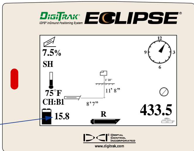
Экран расчетной глубины в режиме локации Eclipse
