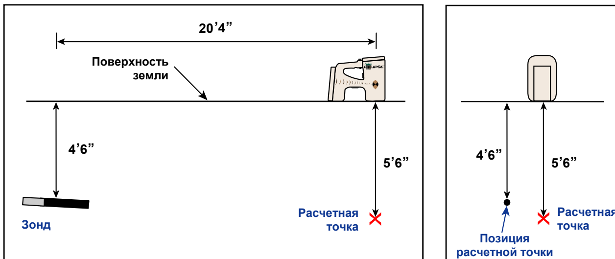
Боковой и фронтальный вид на положение приемника, буровой головки с зондом и расчетной точки
