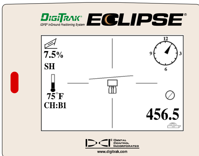
Экран режима локации Eclipse. Приближение приемника к линии локации LL
