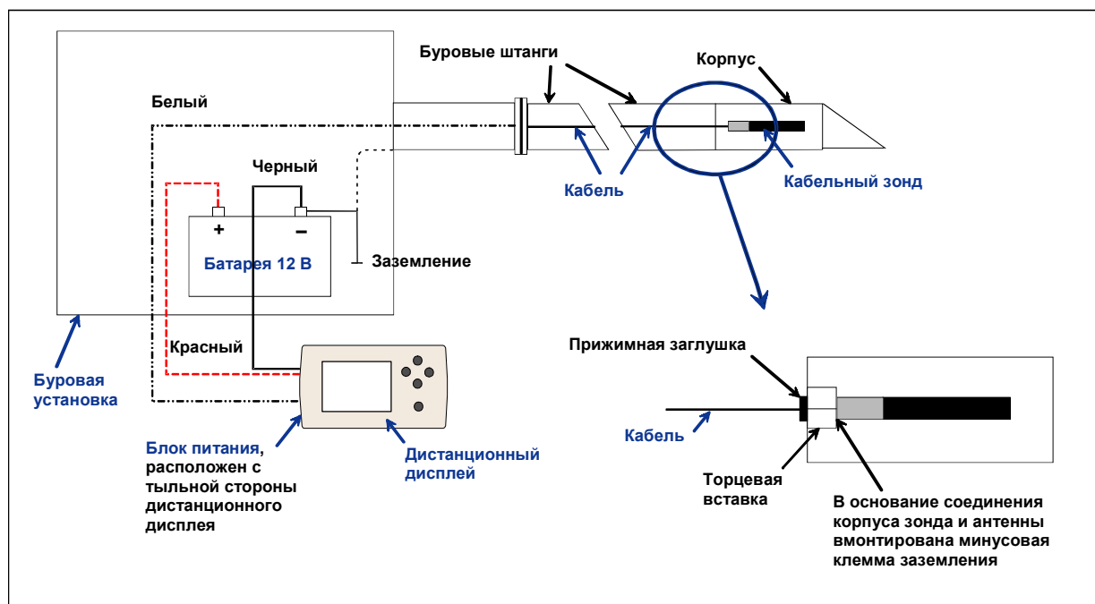
Принципиальная схема соединений компонентов кабельной системы
