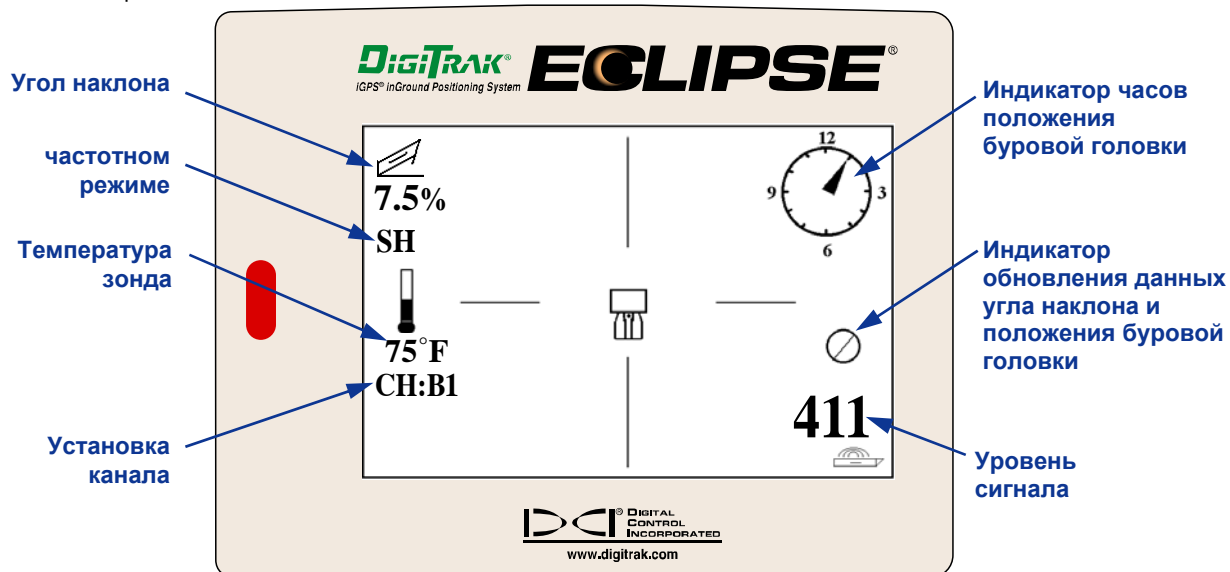
Экран режима локации
