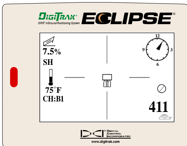
Экран режима локации
