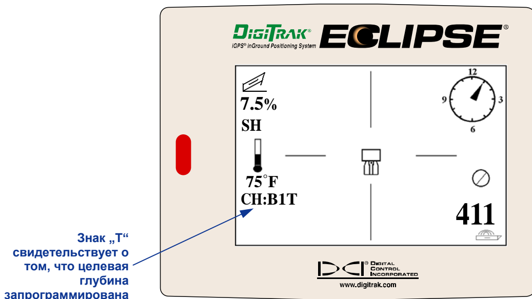
Экран приемника: целевая глубина запрограммирована
