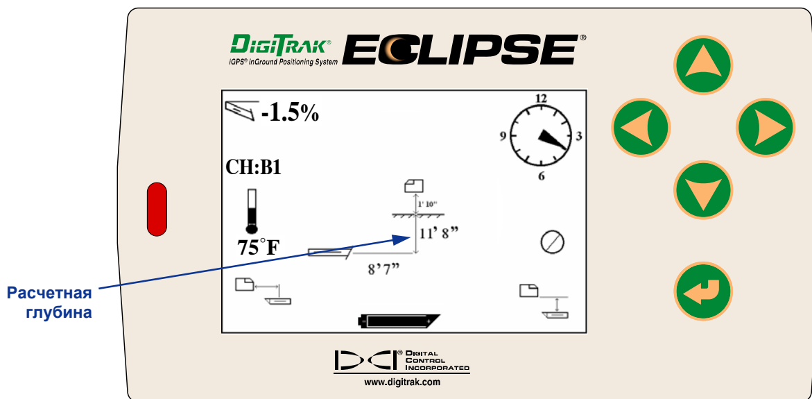
Экран дистанционного дисплея с показанием расчетной глубины (приемник находится над точкой локации FLP или RLP)
