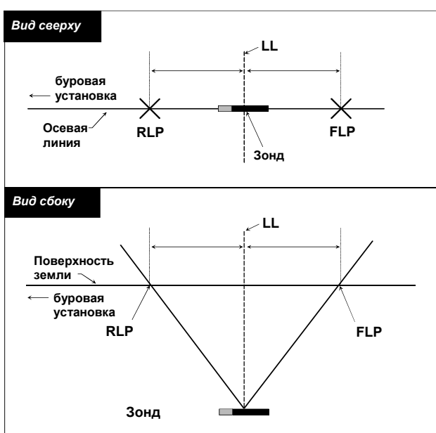
Вид сверху и сбоку на точки FLP или RLP и линию LL, когда зонд расположен параллельно поверхности земли
