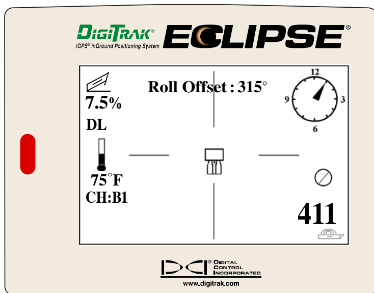
Приёмник Eclipse с указанной на экране величиной угла компенсации
