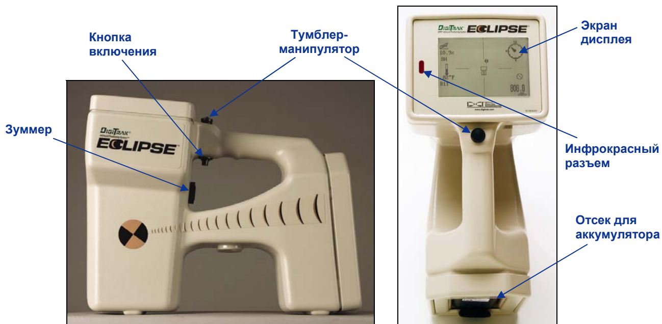
Вид на приемник Eclipse сбоку (см. слева) и вид на приемник сверху (см. справа)
