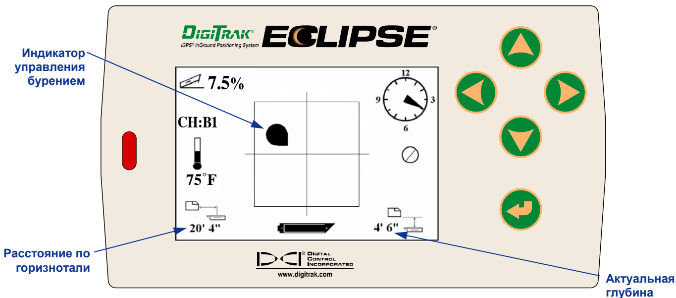
Экран Target Steering на дистанционном дисплее
