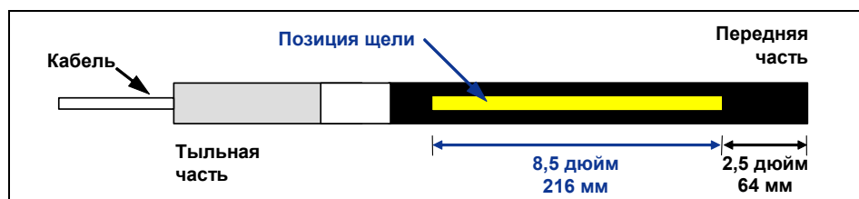
Расположение прорезей на кабельном зонде
