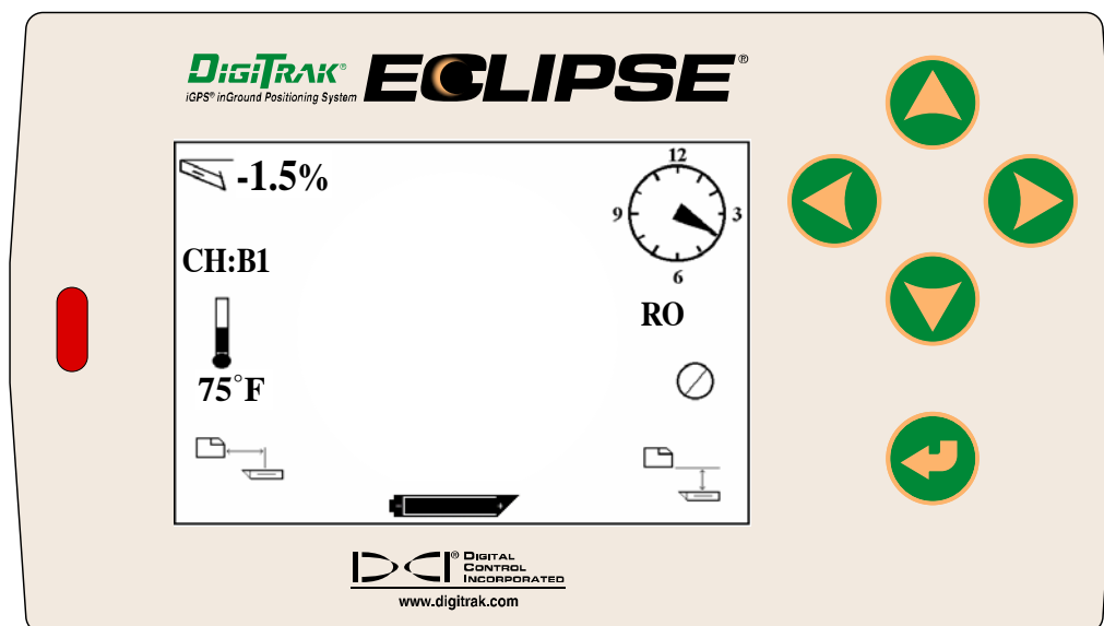
Дистанционный дисплей системы Eclipse с указанным параметром компенсации угла поворота
