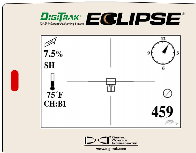
Экран режима локации Eclipse. Приемник находится на линии локации с целевой точкой LL
