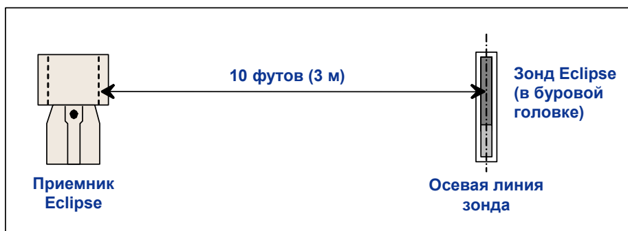
Замер расстояния в 3 м (10 фунтов) для проведения калибровки по одной точке
