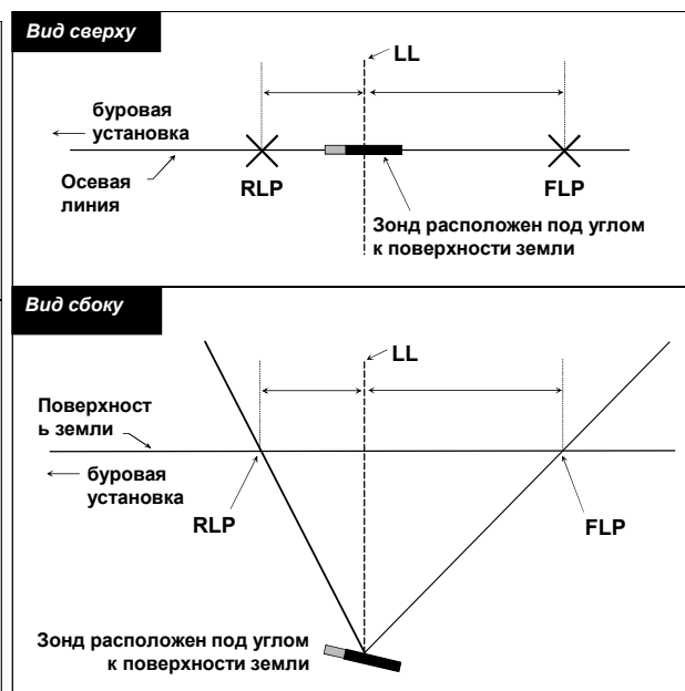
Вид сверху и сбоку на точки FLP или RLP и линию LL, когда зонд расположен под углом к поверхности земли
