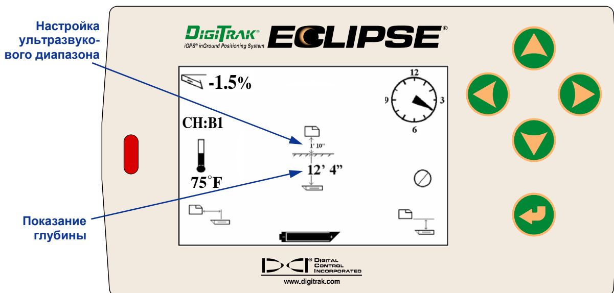
Экран дистанционного дисплея с показанием глубины (приемник находится над линией локации LL)
