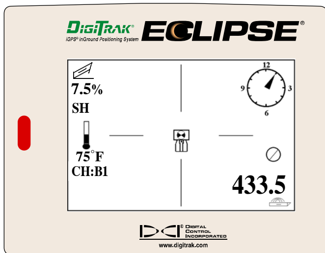
Экран режима локации Eclipse с целевой точкой в приемном окошке над точкой FLP
